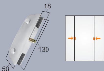
1110 Dobradiça pivotante superior Bisagra pivotante superior
