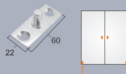
1201-A Pivô p/ dobradiça inferior Pivote para bisagra inferior
