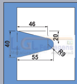
2701, 2702 (colante), 2703, 2704 e 2705
