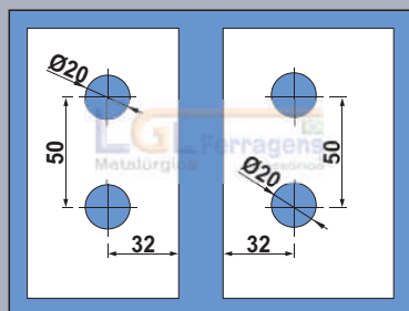
1319 à 135°
