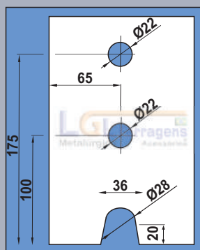
1101 e 1103-Jumbo
