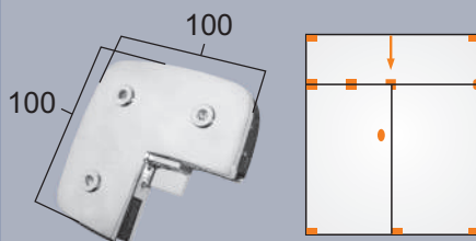
1315 Suporte p/ união de dois ou três vidros em "L" com batedor Soporte para unión de dos o tres vidrio en "L" con batedor
