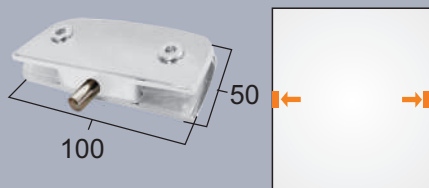
1130 Suporte p/ basculante e pivotante com pino Soporte para basculante y pivotante con pin
