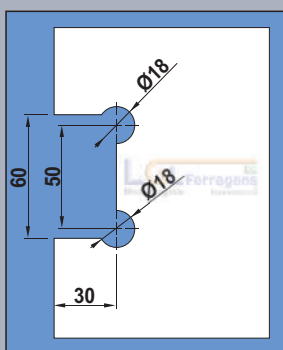
1120 e 1121
