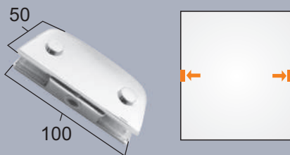
1231 Suporte com ponto de giro p/ basculante e pivotante Soporte con punto de giro para basculante y pivotante
