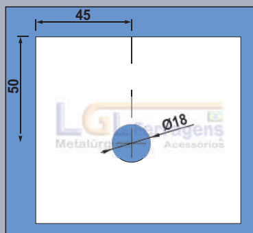
1335 Guia embutida
