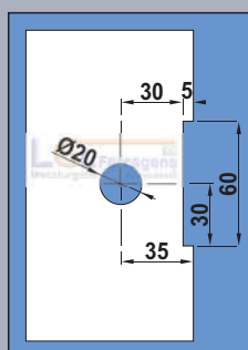
1136 e 1136-B
