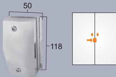
3211 Contra fechadura com batedor p/ 3210 Contra cerradura con batedor para 3210
