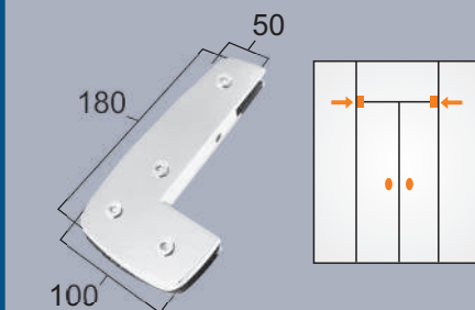
1209 Facão simples lateral e bandeira Machete simple lateral y bandera
