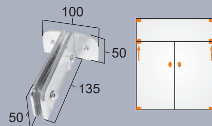
1203 Suporte p/ bandeira com ponto de giro p/ dobradiça superior 1101 Soporte para bandera con punto de giro para bisagra superior 1101
