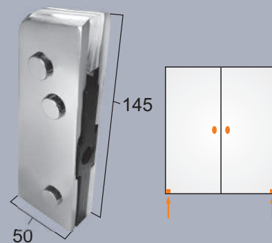
1103-A Dobradiça inferior Bisagra inferior
