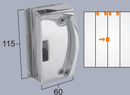
3536-90° Contra fechadura p/ janela de correr Contra cerradura para ventana de corredera
