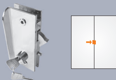
1510 Fechadura bico de papagaio com abas Cerradura pico de loro con pestañas
