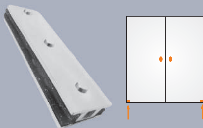
1103 Jumbo | Dobradiça inferior especial Jumbo | Bisagra inferior especial
