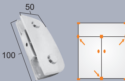
1306 Suporte com miolo p/ união Soporte con núcleo para unión
