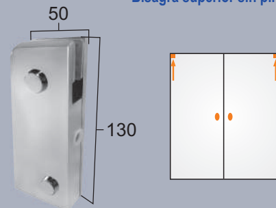
1101-A Dobradiça superior sem pino Bisagra superior sin pin
