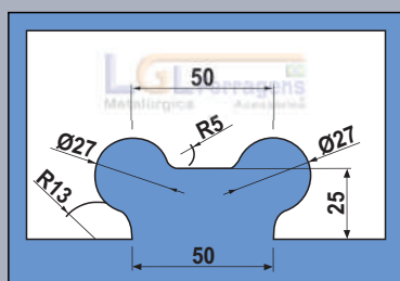
1007 e 1008
