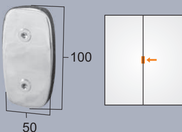
1310 Suporte p/ união de dois ou três vidros em "L" Soporte para unión de dos o tres vidrio en "L"
