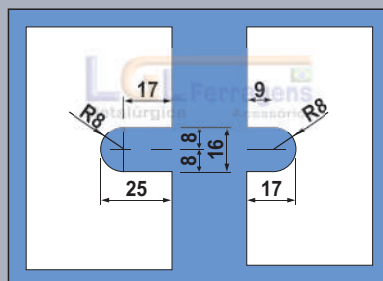
1322 e 3730
